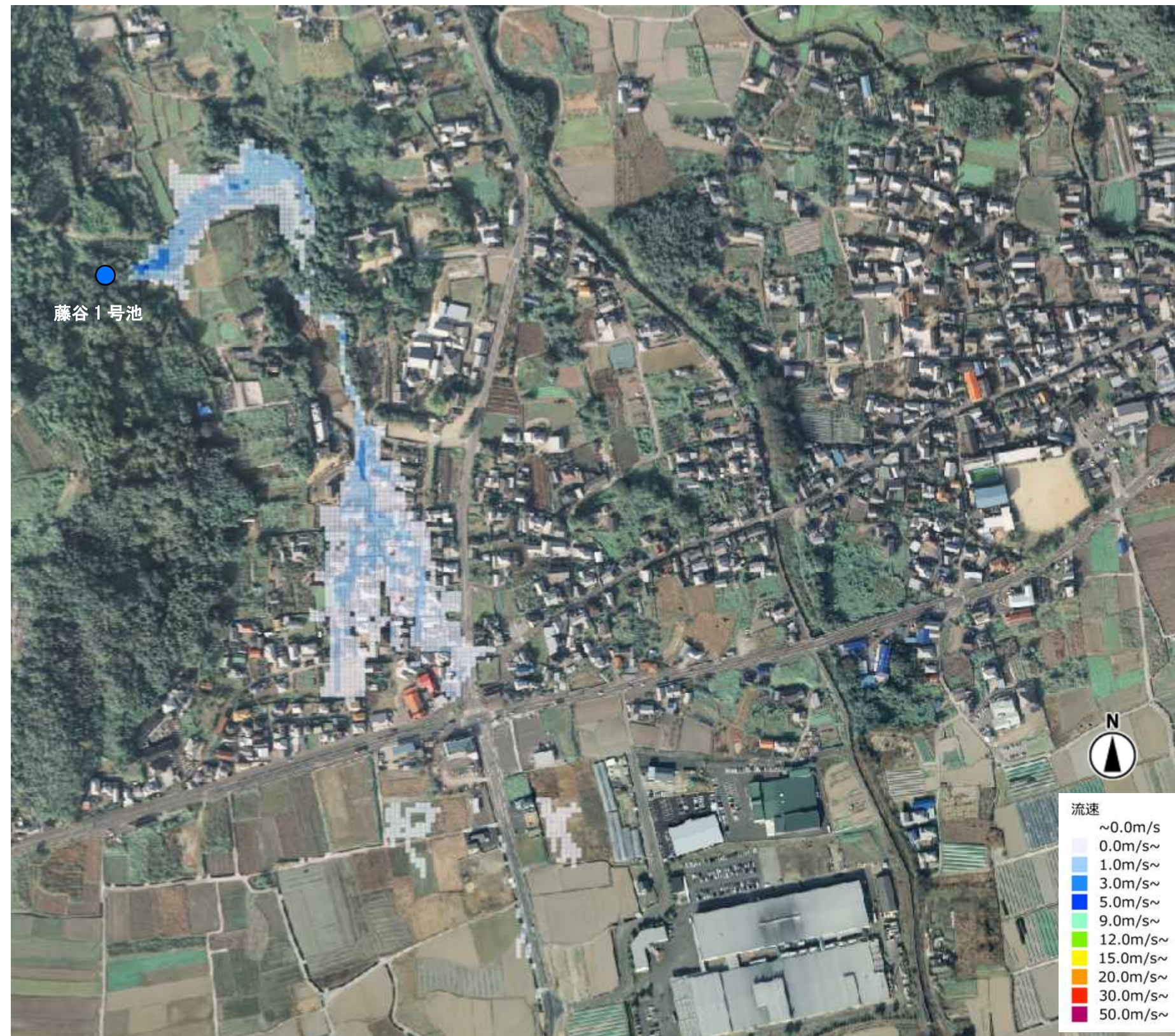
最大流速(藤谷 1号池)
