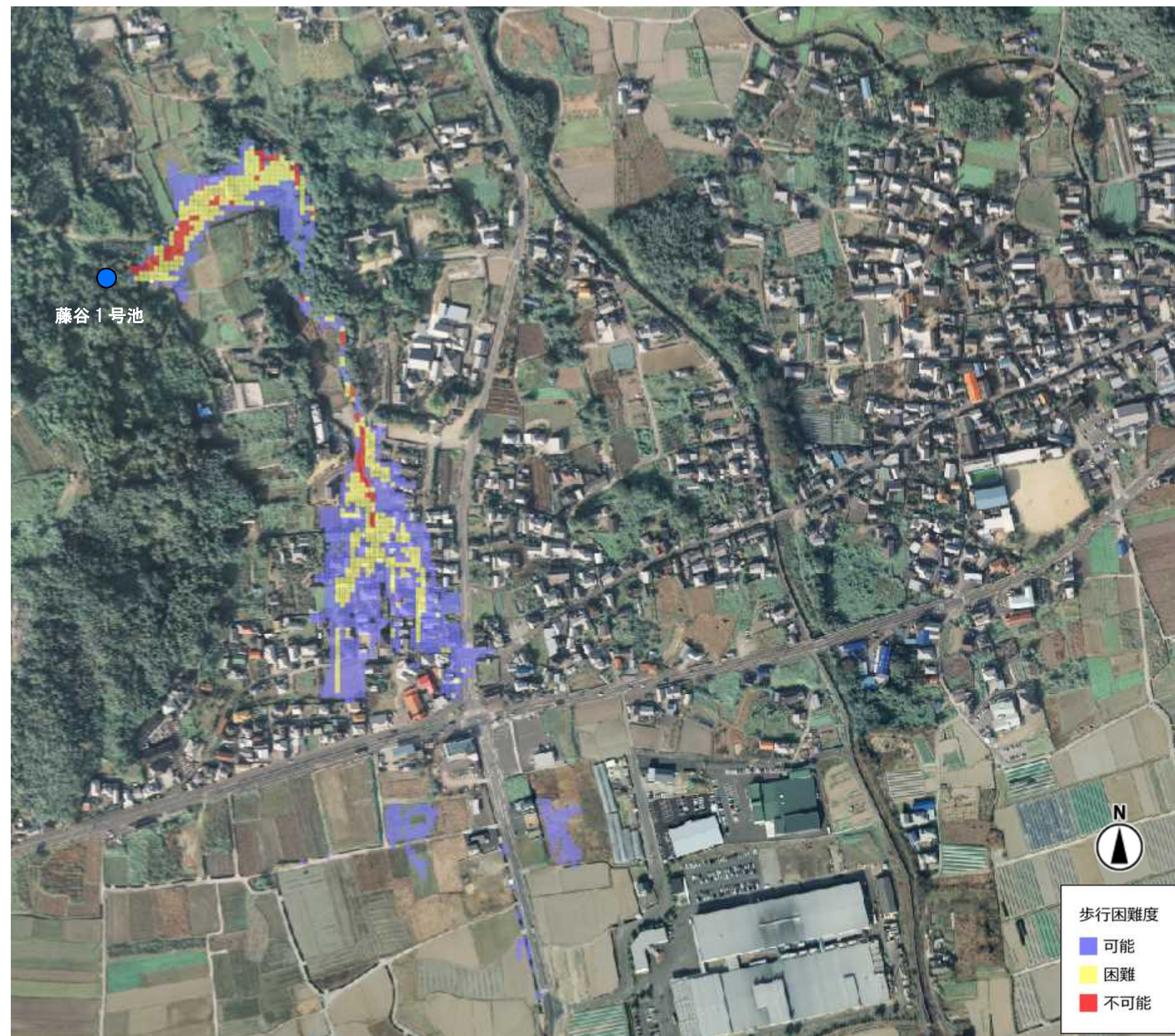
最大歩行困難度(藤谷 1 号池)
