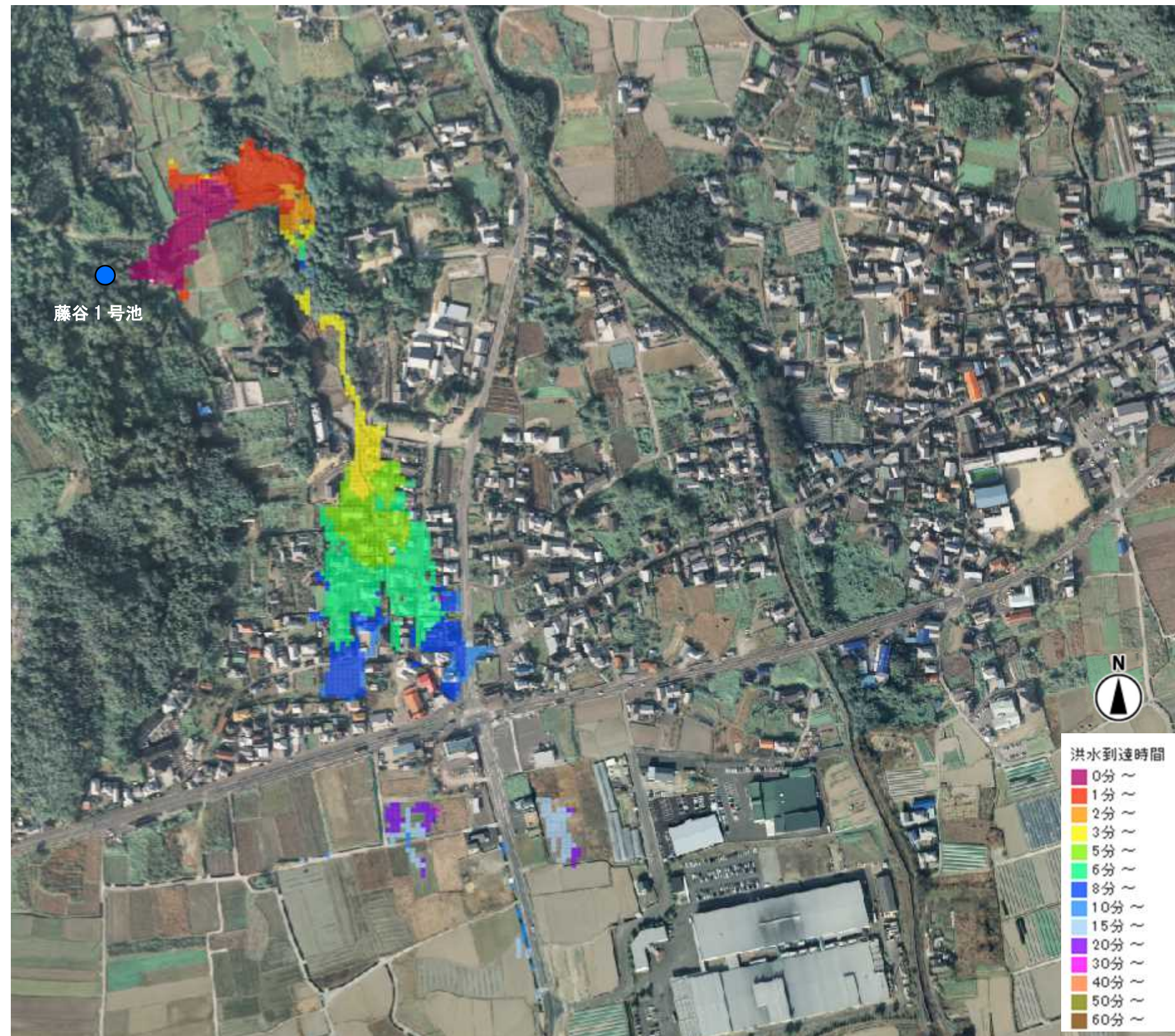
洪水到達時間(藤谷 1 号池)
