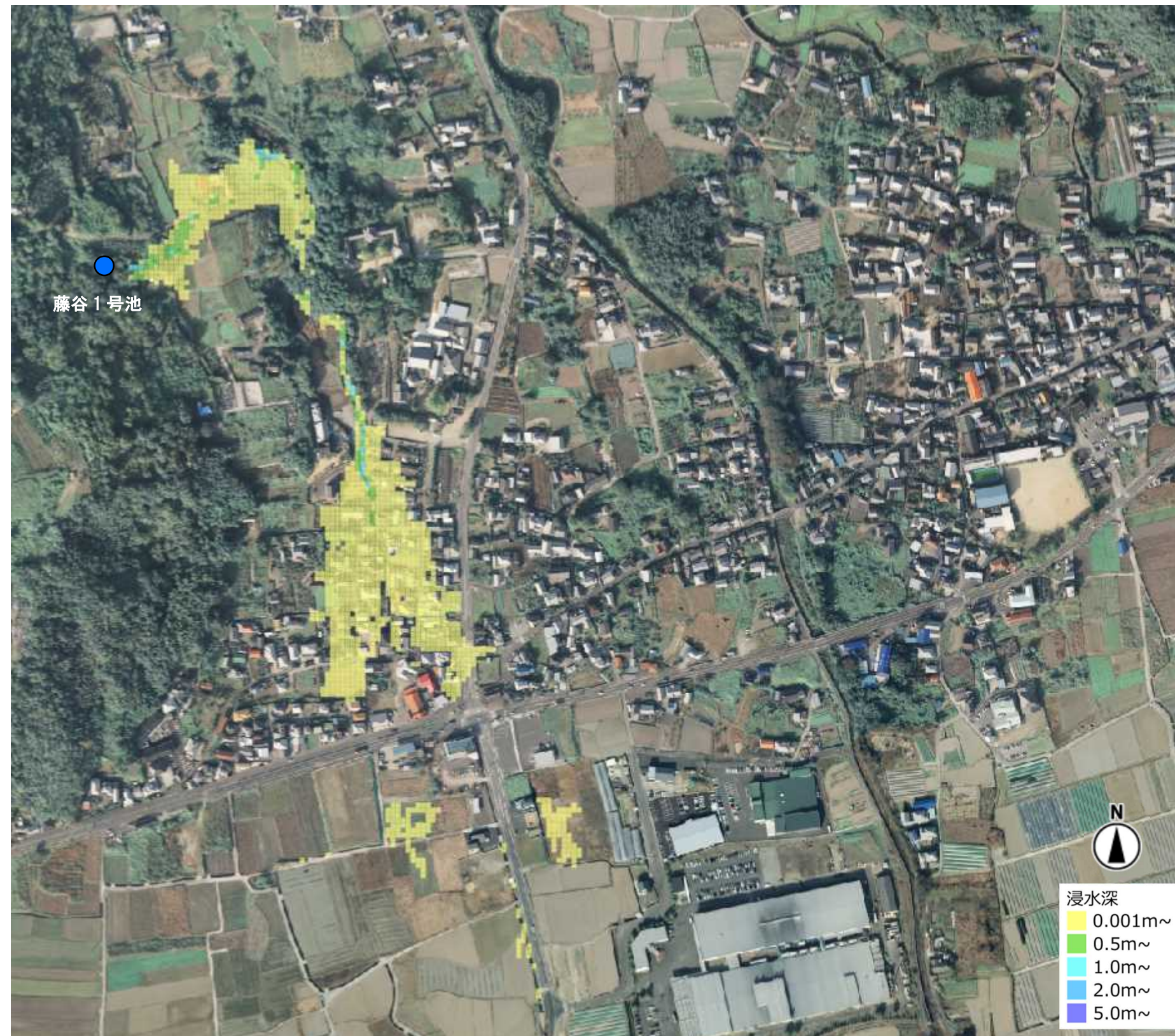
最大浸水深(藤谷 1 号池)
