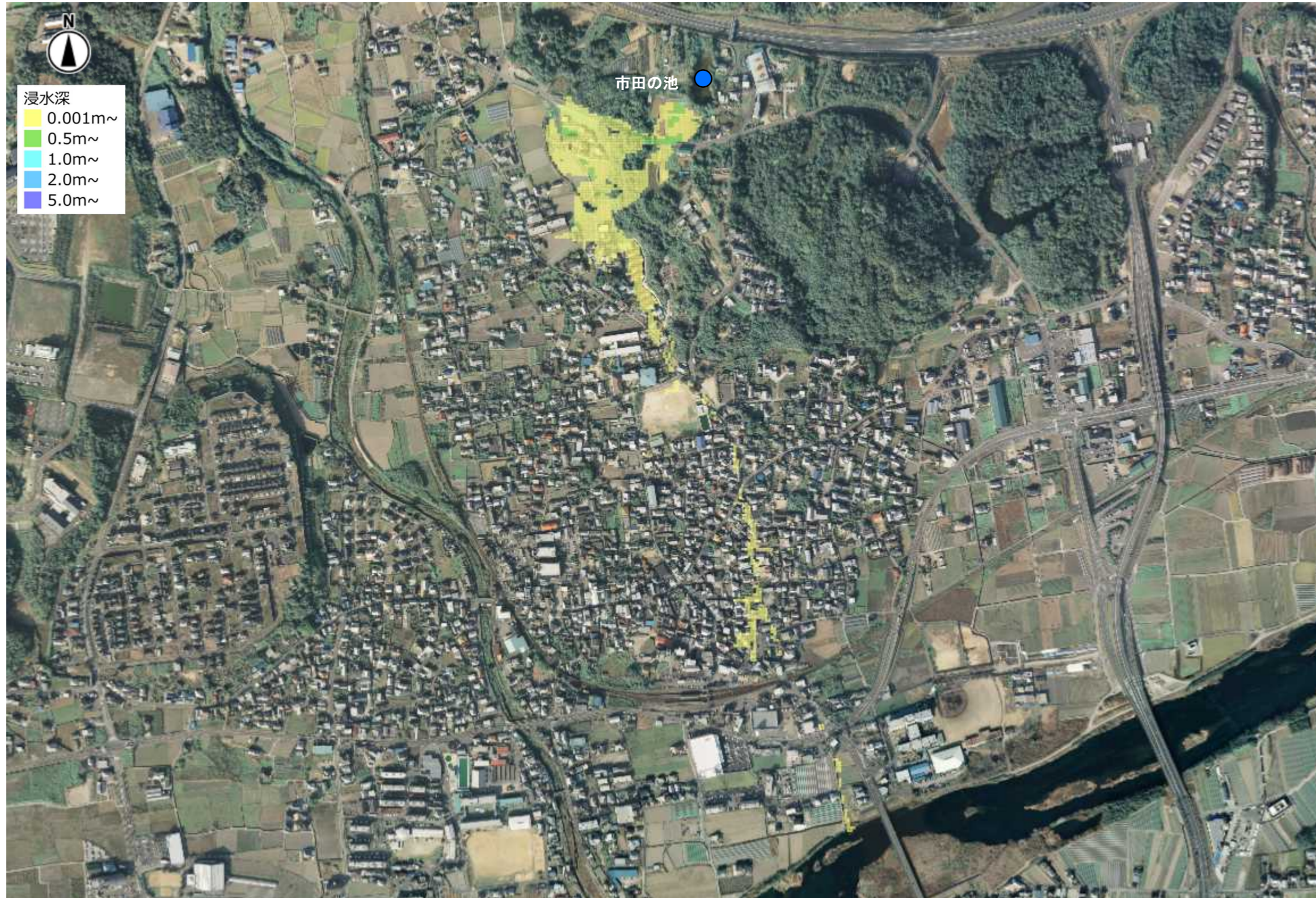
最大浸水深(市田の池)
