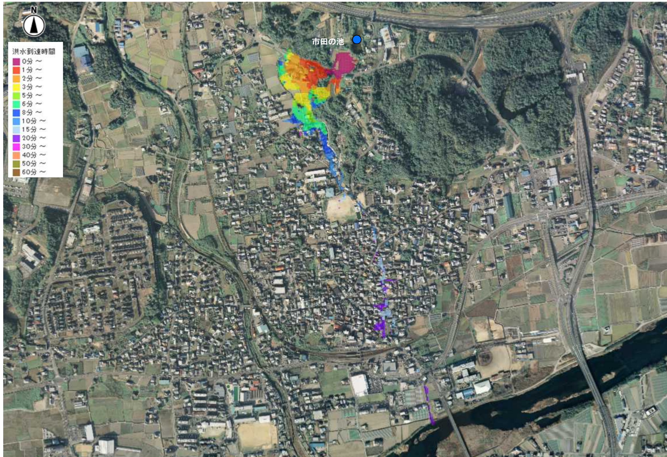
洪水到達時間(市田の池)
