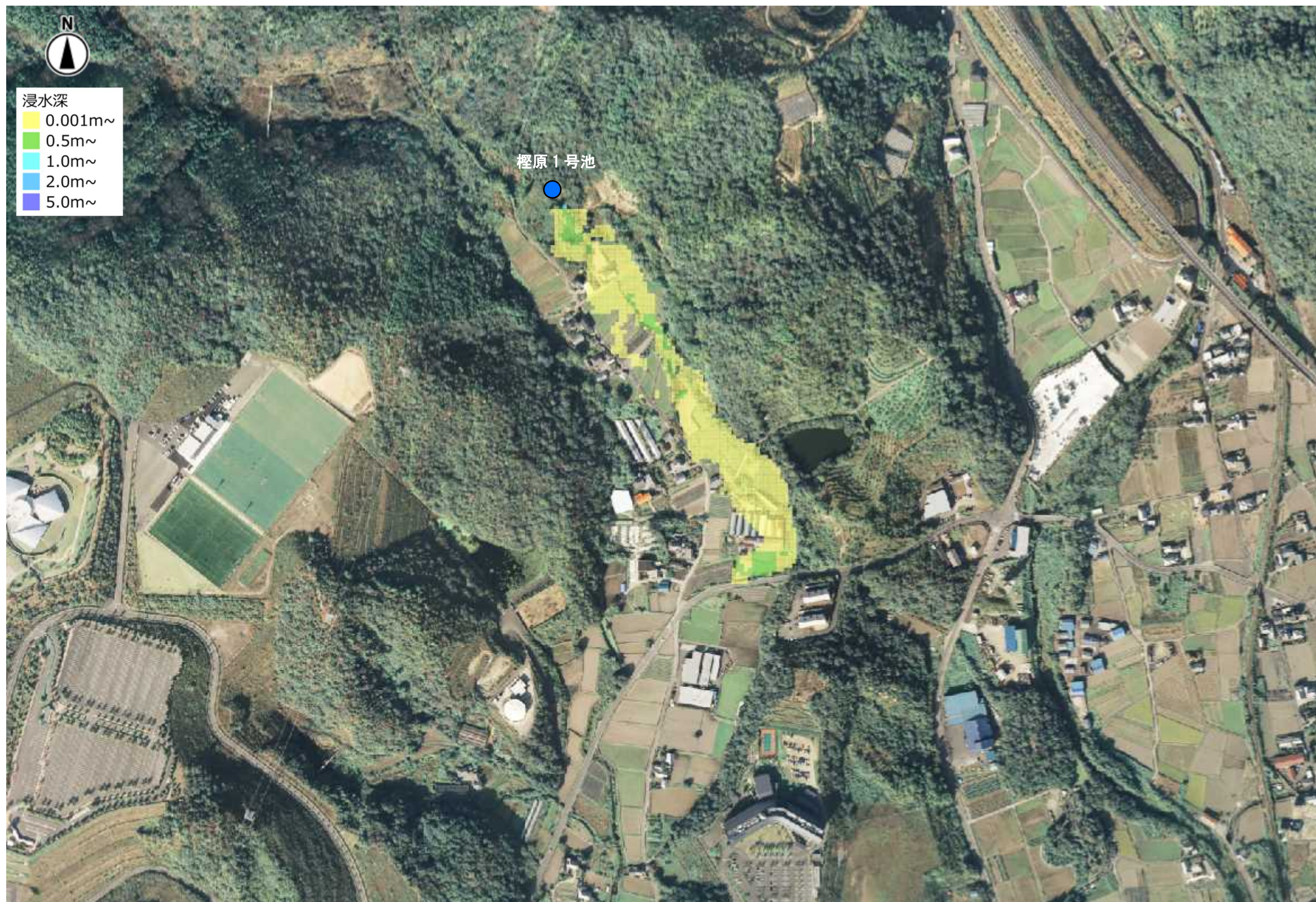
最大浸水深(檜原 1 号池)
