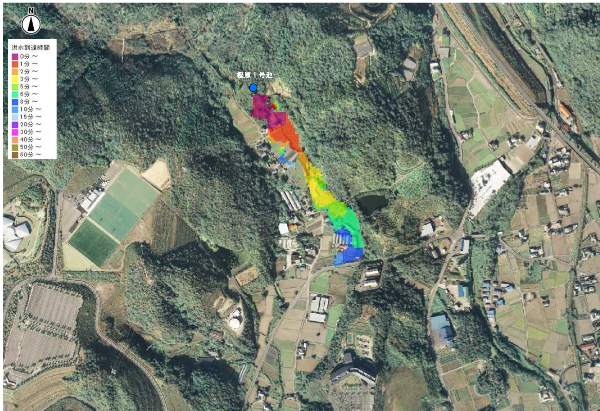
洪水到達時間(檜原1号池)
