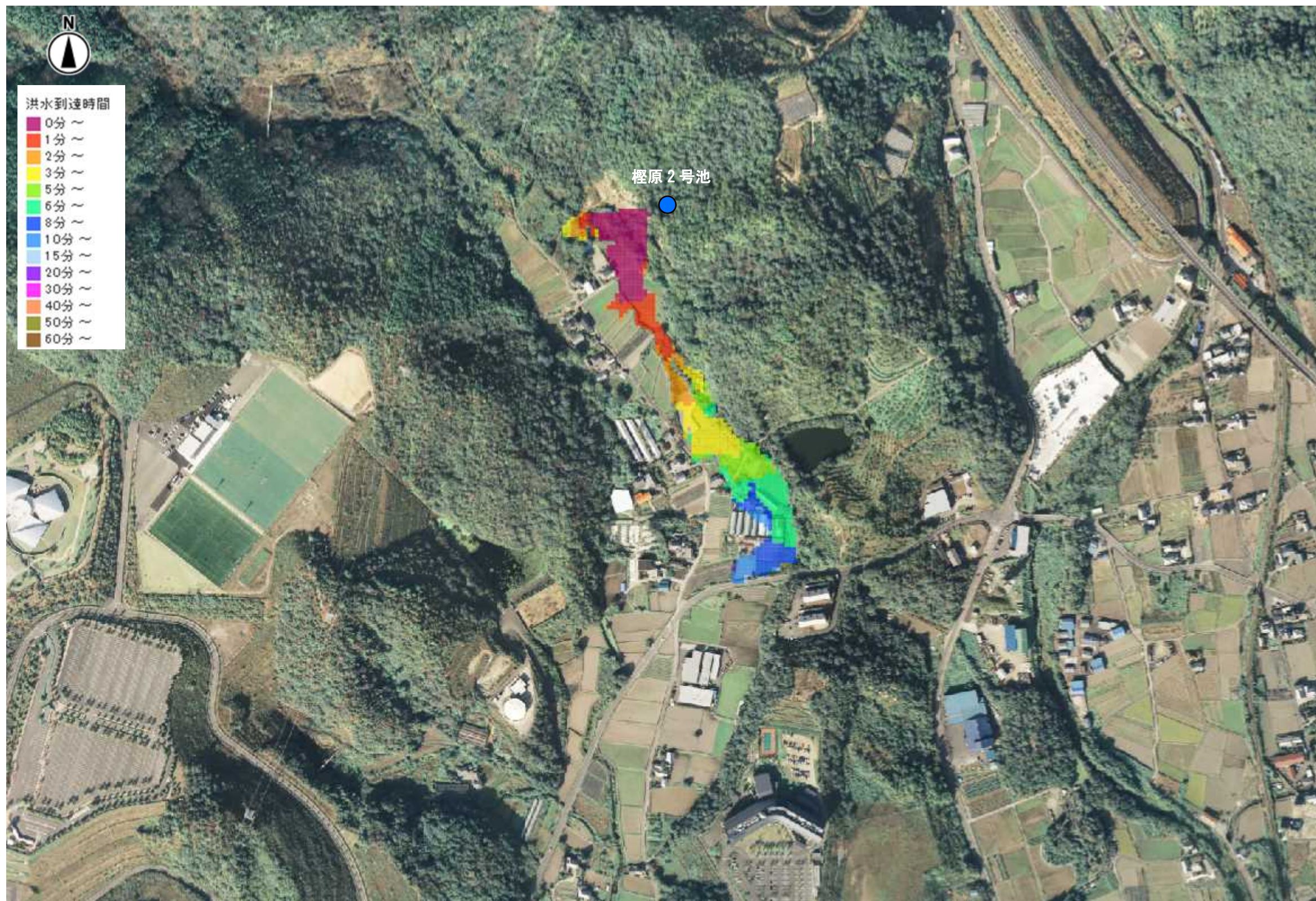
洪水到達時間(檜原 2 号池)
