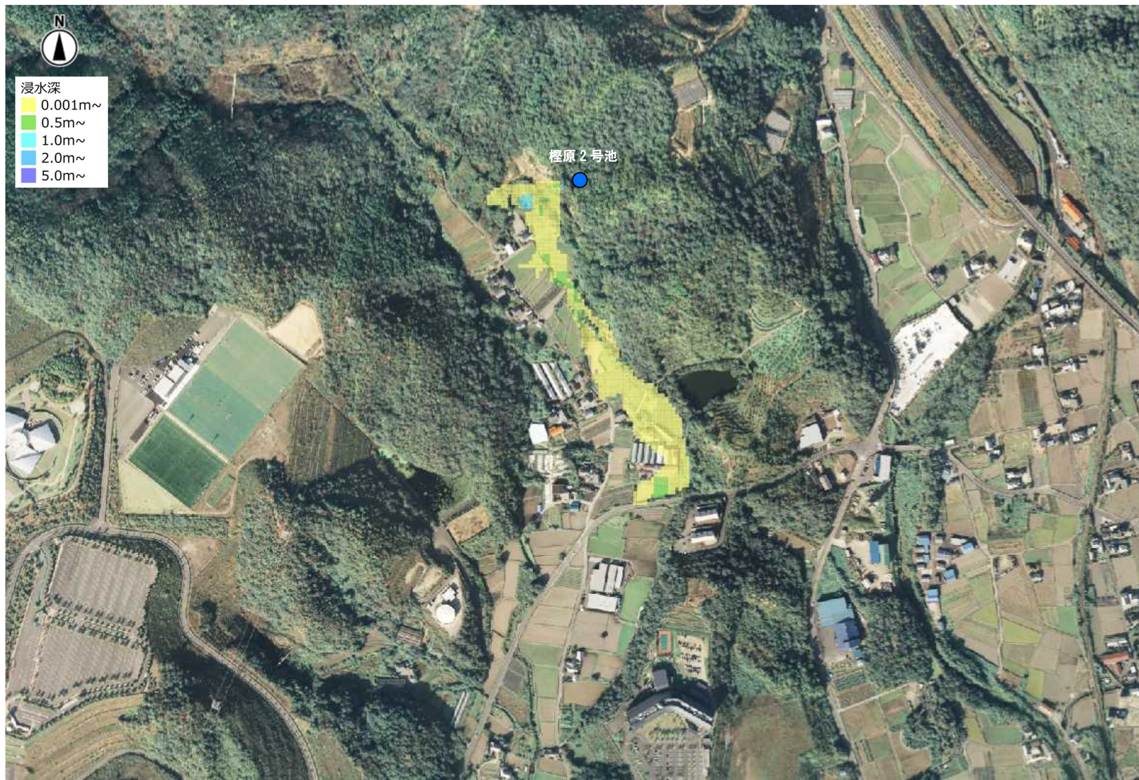
最大浸水深(檜原 2 号池)
