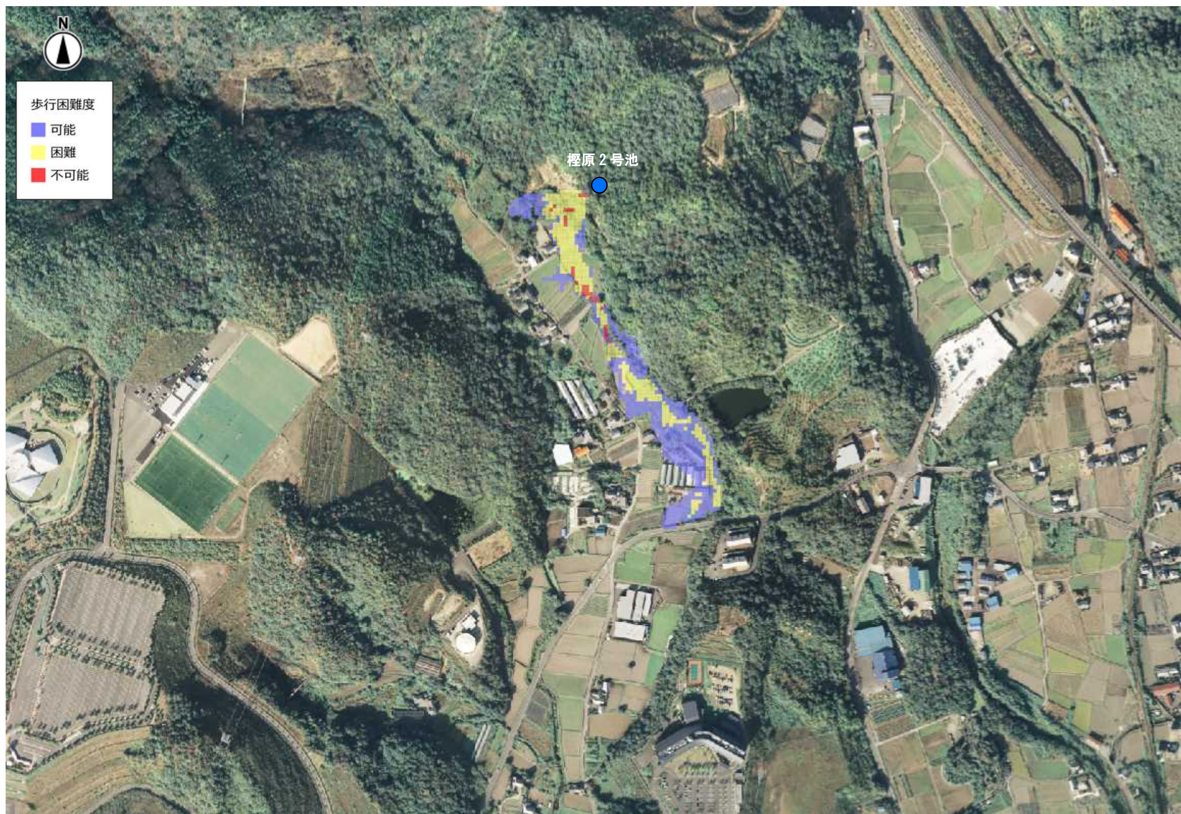
最大歩行困難度(桧原 2号池)
