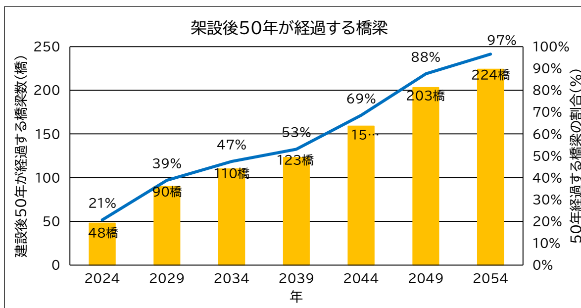
図- 建設から50年以上が経過した橋梁の割合の推移
